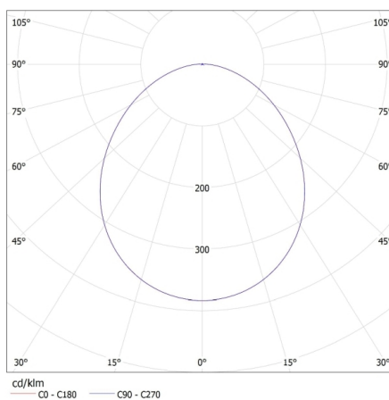
KANLUX S.A. (kat 22700) TOMI LED5W GU10-WW / Krzywa rozsyłu światła (biegunowo)
